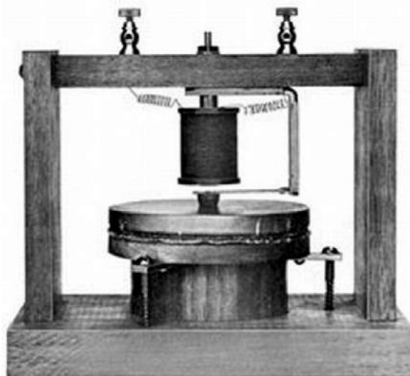
Перша діюча модель телефону Белла.
