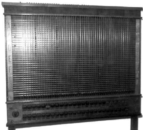
Дошка Гіллеланда на 50 номерів.
