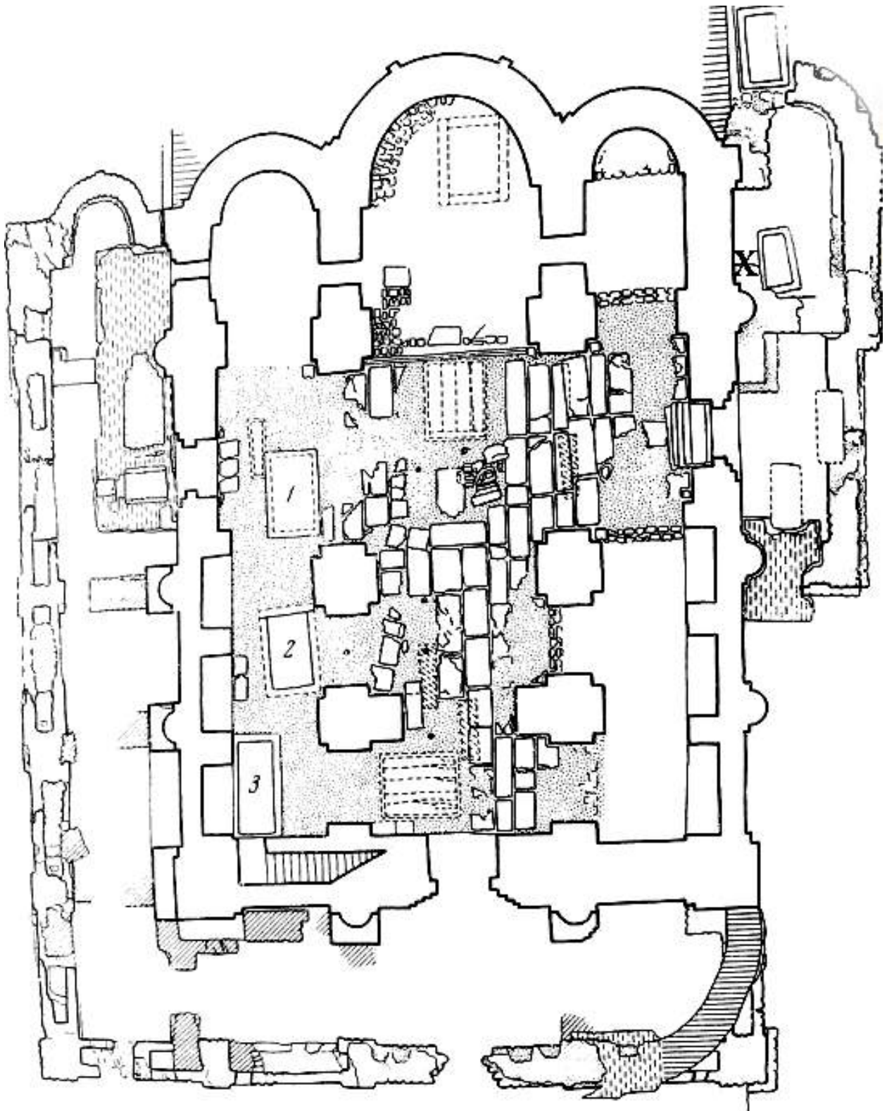
Рис. 1. Борисоглібський собор. План М.В. Холостенка.
